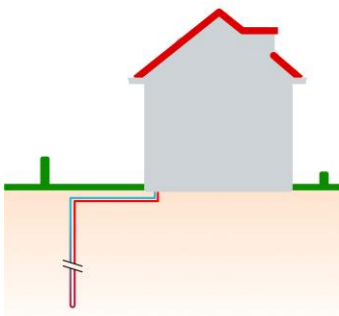
Figuur 3 Schematische weergave van een gesloten bron
